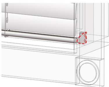
MONTAJE INTERIOR - Soporte de sujeción
