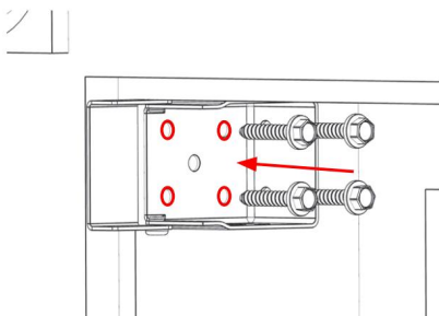
Requisitos de profundidad de montaje interior
